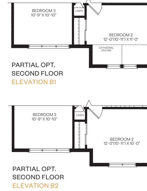
ELEVATION B
